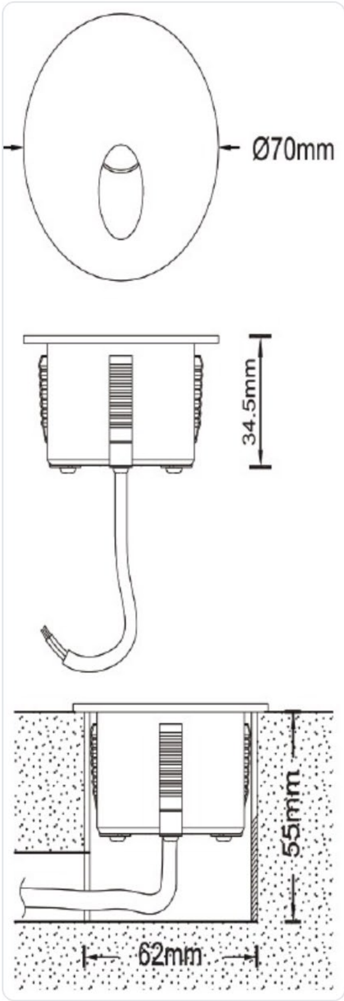
Ø 70 mm en surface — encastrement Ø 62 × 55 mm
