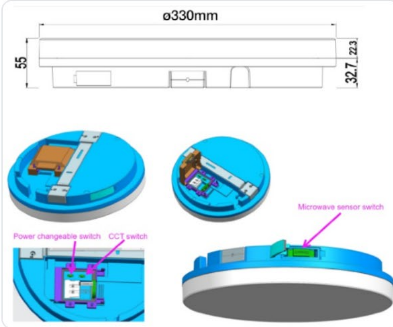
Dimensions, interrupteurs puissance / CCT & capteur HF
